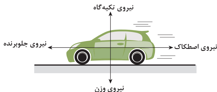
شکل ۱۰-۲ تعدادل دینامیکی خودرو
