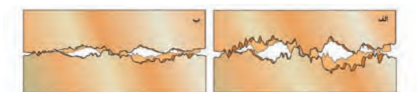
شکل ۲-۲۶ این شکل تأثیر نیروی عمودی تکیه‌گاه بر نیروی اصطکاک را نشان می‌دهد. در شکل الف نیروی عمودی تکیه‌گاه کمتر از شکل ب است و سطح تماس در مقیاس ریز کمتر بوده و نیروی اصطکاک کمتر است.
