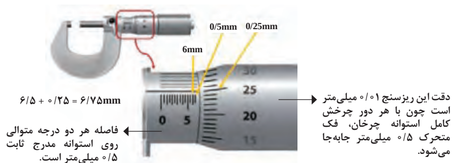
شکل ۱-۱۴ نحوه خواندن نتیجه اندازه‌گیری با ریزسنج ۰/۰۱ میلی‌متری
