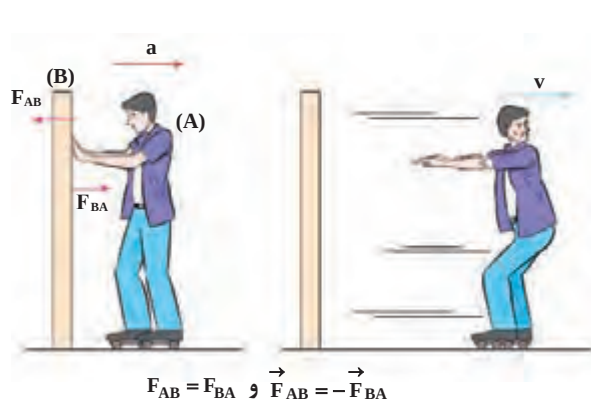
شکل ۲۰-۲ حرکت اسکیت باز به عقب بر اثر نیروی واکنش دیوار
